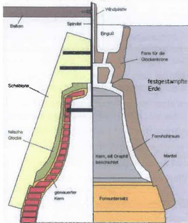
Schnitt durch eine Glockenform: links bei der Formherstellung, rechts die in einer Formkasten oder Gießgrube eingesetzte Form vor dem Gieß
